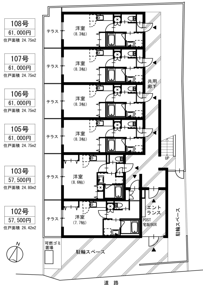
配置図兼 1 階平面図
