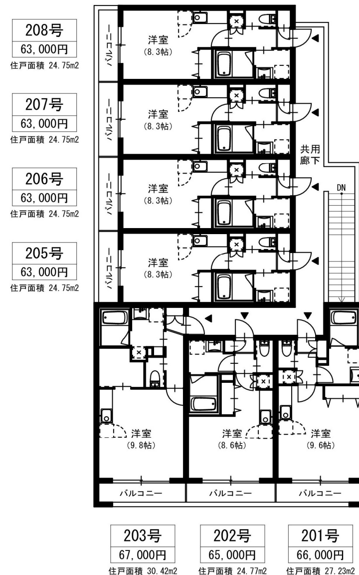
2 階平面図
